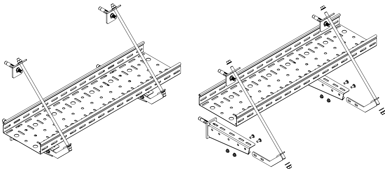
Крепление к стене с лотком и с КРН5
